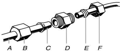
A. Tubería de agua B. Tuerca (provista) C. Bulbo D. Acoplamiento (provisto) E. Férula (adquirida) F. Tuerca (adquirida)
